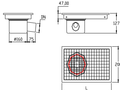
Eğimsiz - Yandan Çıkışlı - Kenardan Sifonlu Çıkış Ölçüsü DN 50 - DN 70
