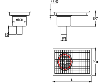
Eğimsiz - Alttan Çıkışlı - Kenardan Sifonlu Çıkış Ölçüsü DN 50 - DN 70
