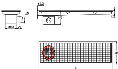
Bir Yöne Eğimli - Yandan Çıkışlı - Kenardan Sifonlu Çıkış Ölçüsü DN 50 - DN 70
