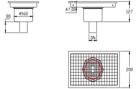
Eğimsiz - Alttan Çıkışlı - Ortadan Sifonlu Çıkış Ölçüsü DN 50 - DN 70
