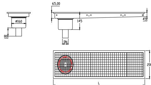
Bir Yöne Eğimli - Alttan Çıkışlı - Kenardan Sifonlu Çıkış Ölçüsü DN 50 - DN 70
