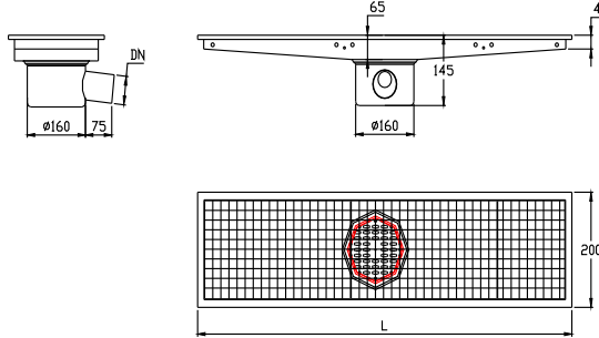
Ortaya Eğimli - Yandan Çıkışlı - Ortadan Sifonlu Çıkış Ölçüsü DN 50 - DN 70
