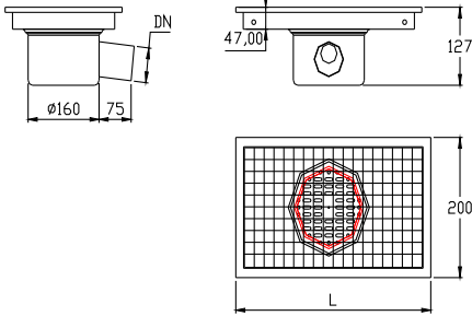
Eğimsiz - Yandan Çıkışlı - Ortadan Sifonlu Çıkış Ölçüsü DN 50 - DN 70
