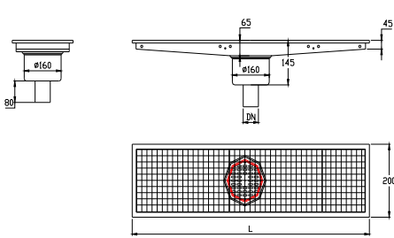
Ortaya Eğimli - Alttan Çıkışlı - Ortadan Sifonlu Çıkış Ölçüsü DN 50 - DN 70
